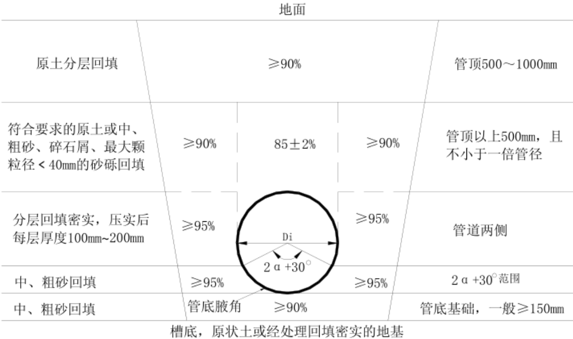
图 4.6.3 柔性管道沟槽回填部位与压实度示意图
