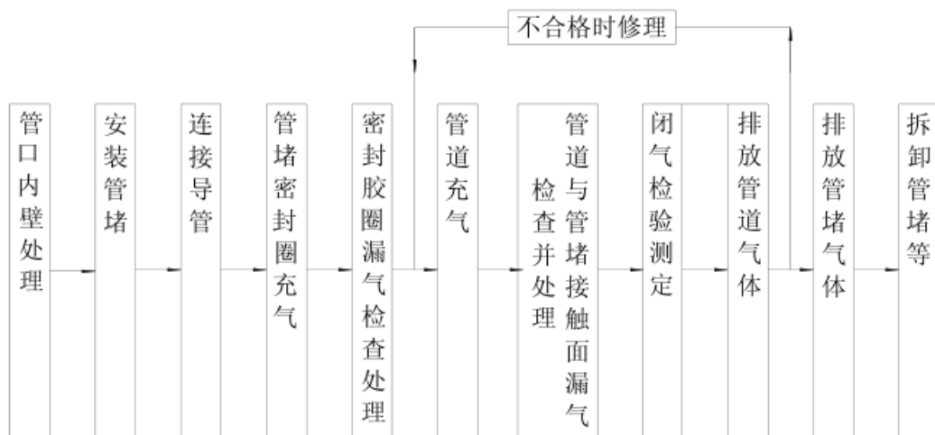
图 E. 0. 2 管道闭气检验工艺流程图
