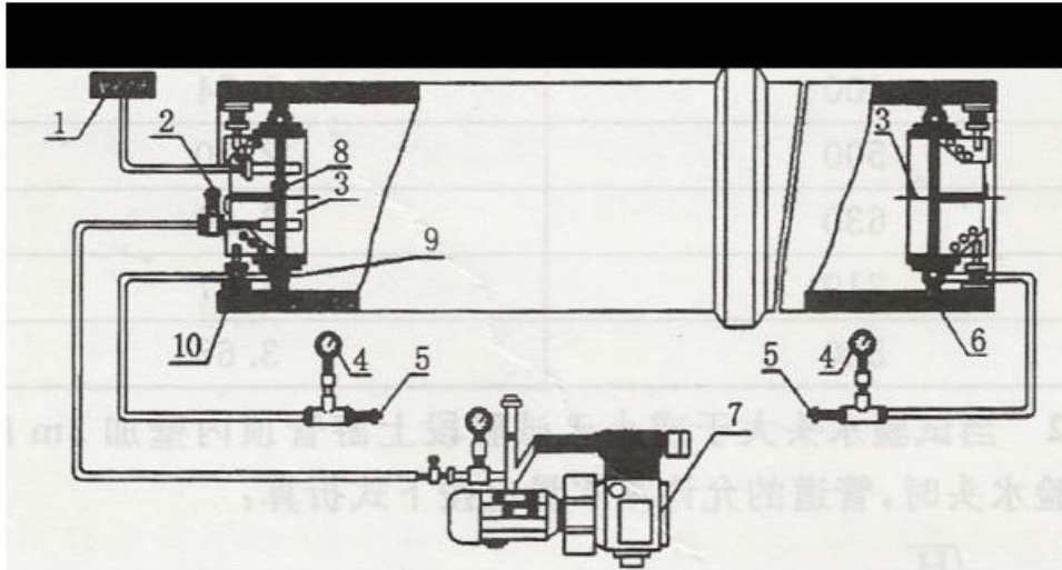
图 E.0.1 排水管道闭气检验装置图
