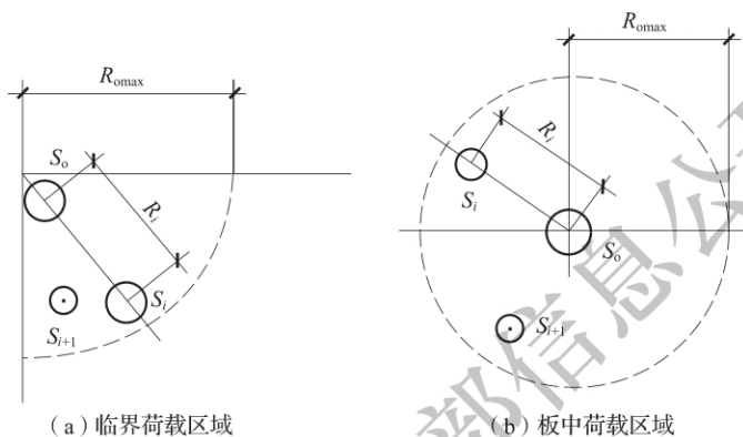
图 C. 2. 9 荷载区域
